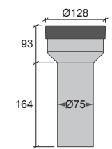
E + K3 WC - Stos 75, Centrisk RSK 310 67 22
