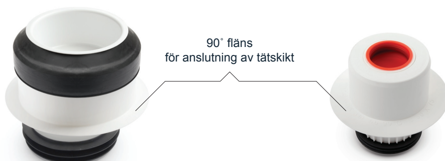
Exempel på WC - stös
