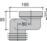
A + K2 WC - Stos Offset 80, Excentrisk 80 mm RSK 310 66 79 NRF 619 66 54
