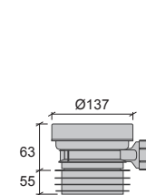
A + K1 WC - Stos, X-tra, Centrisk RSK 310 66 64 NRF 619 66 73
