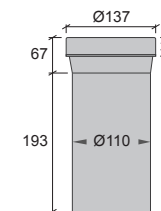
C + K3 WC - Stos 110 muff Centrisk RSK 310 66 86
