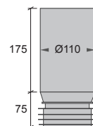
A Rörförlängare Centrisk RSK 310 67 07
