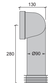
A + K3 WC - Stos, Universal RSK 310 67 20 NRF 619 66 71
