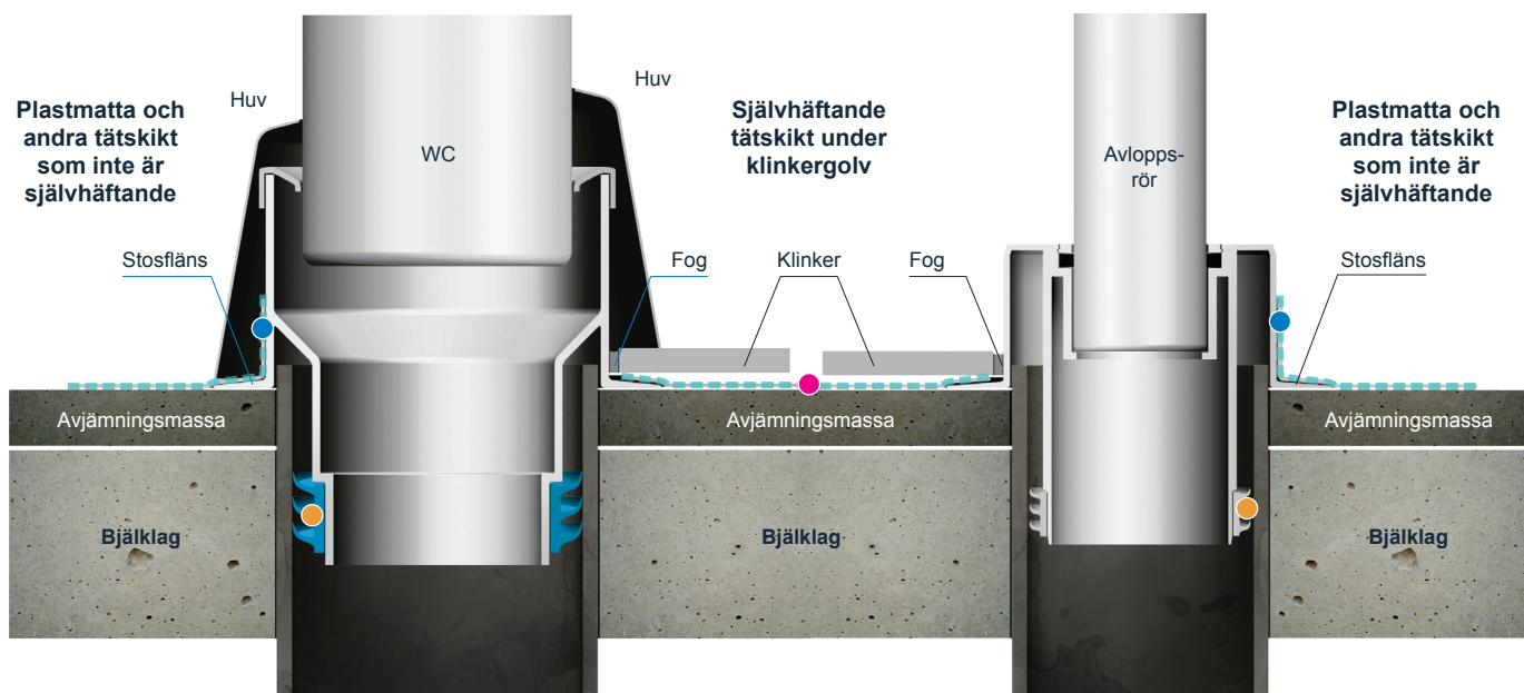
Exempel på golvanslutningsstos (GAS)
